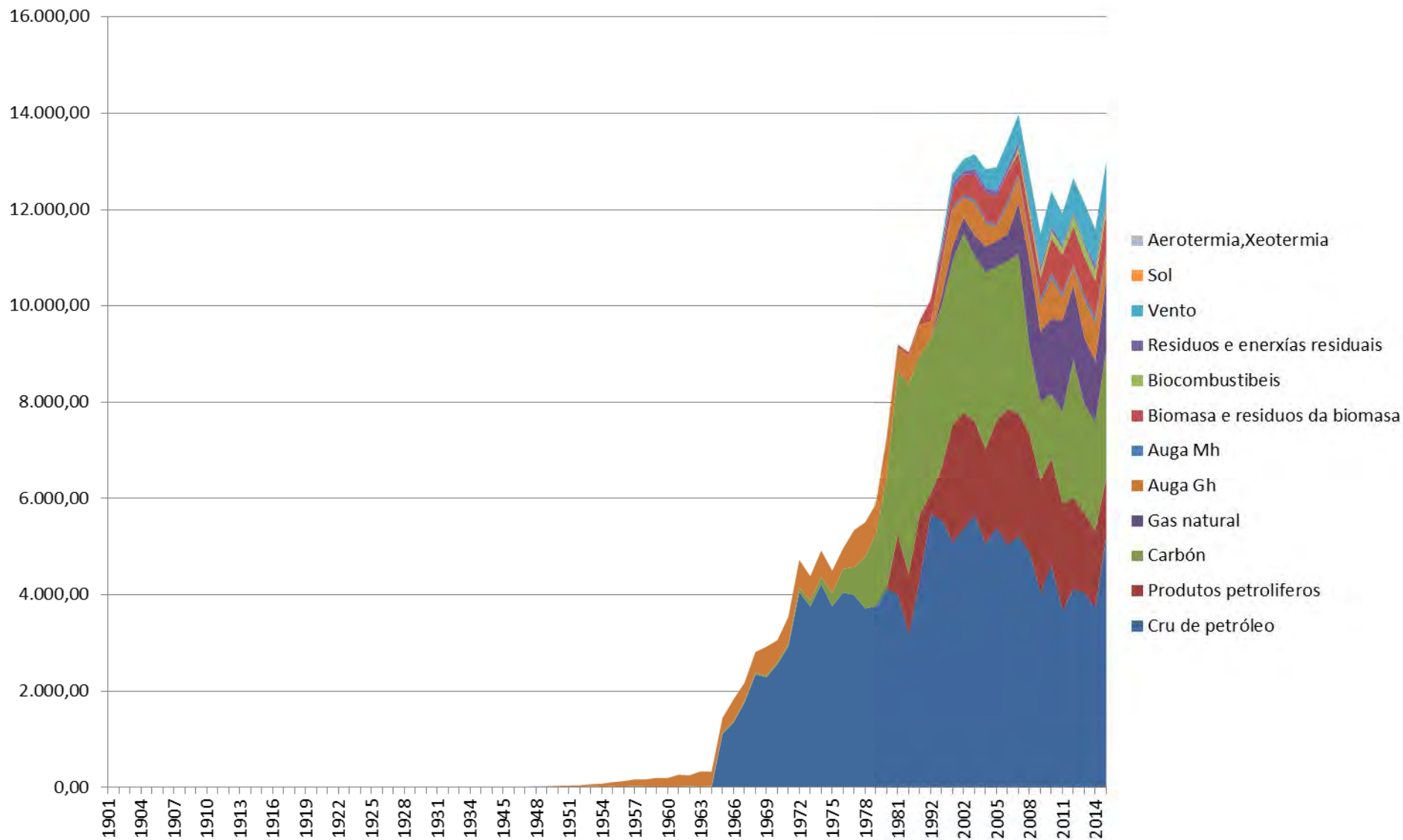
Gráfico 2. Evolución da enerxía primaria transformada. Galiza, 1901-2015 (ktep) por fontes
