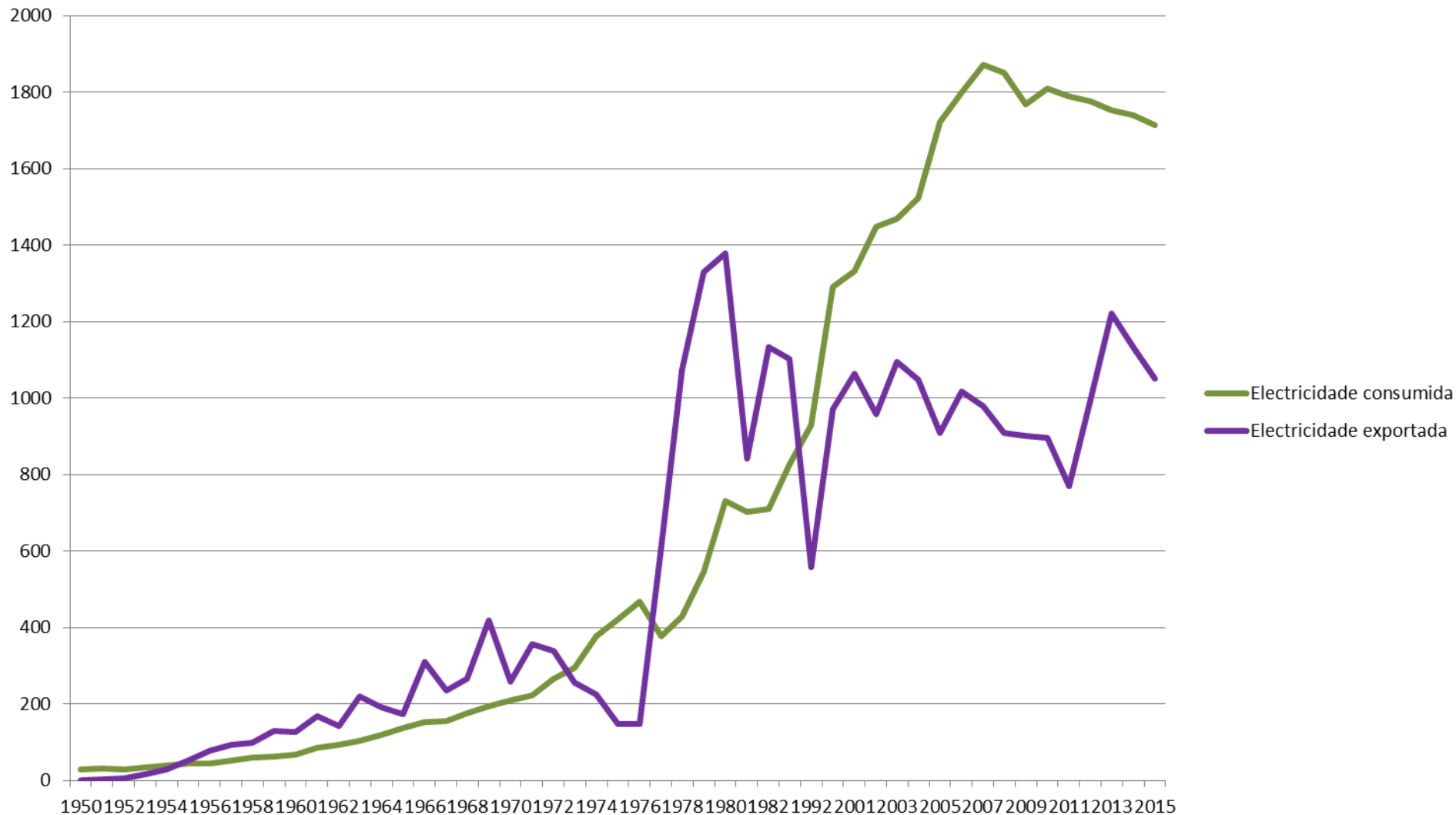
Gráfico 5. Evolución da electricidade consumida en Galiza e da exportada. Galiza, 1950-2015 (ktep)
