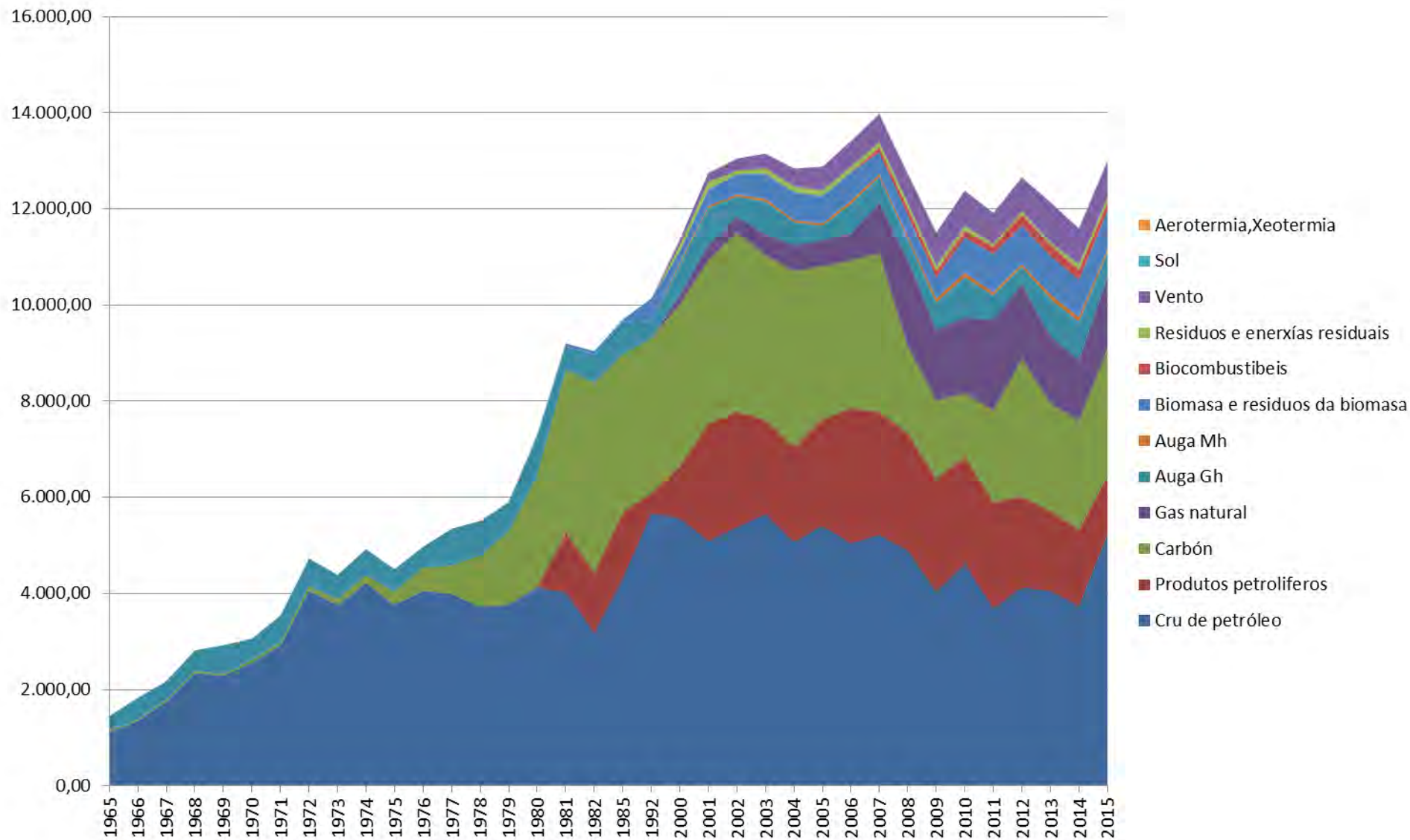
Gráfico 11. Evolución dos distintos tipos de enerxía primaria. Galiza, 1965-2015 (ktep)
