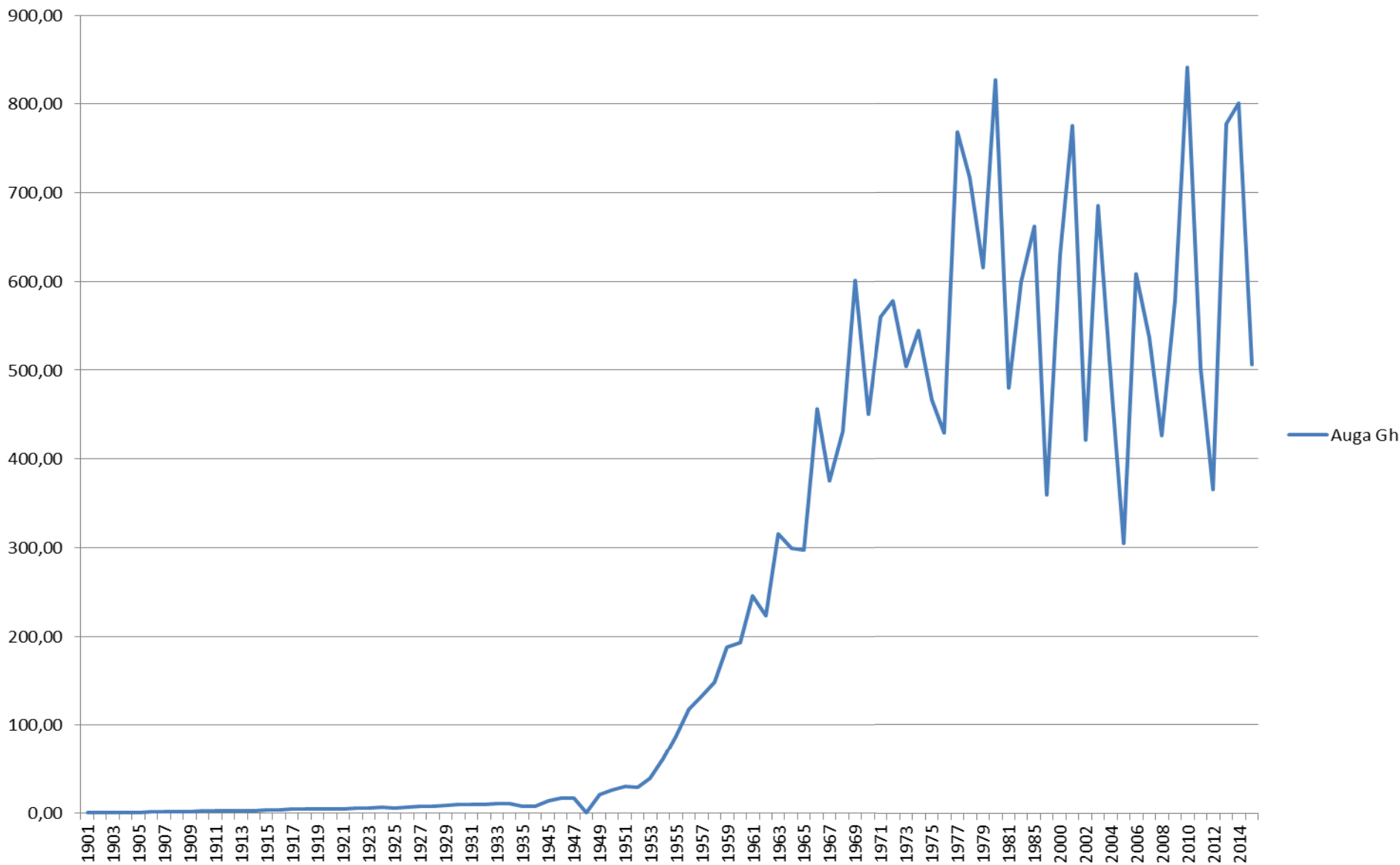
Gráfico 6. Evolución da produción de enerxía hidráulica. Galiza, 1901-2015 (ktep)
